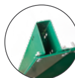
Palo Omega con piatto 60x40x25x3 o 120x60x30x3 mm
